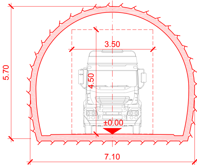
Sección A-A Galería de acceso/salida principal
