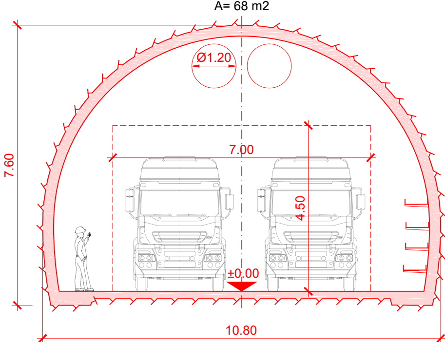
Sección B-B Galería de conexión interna Laboratorio
