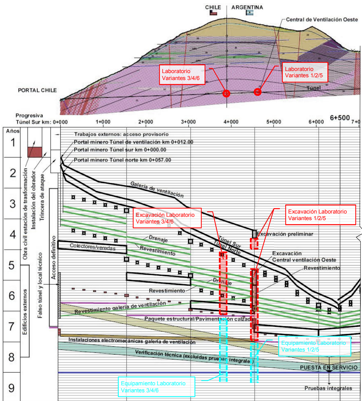
Figura 2: Extracto del cronograma preliminar del TAN con trabajos Laboratorio
