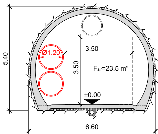
Sección D-D Galería de conexión interna Laboratorio
