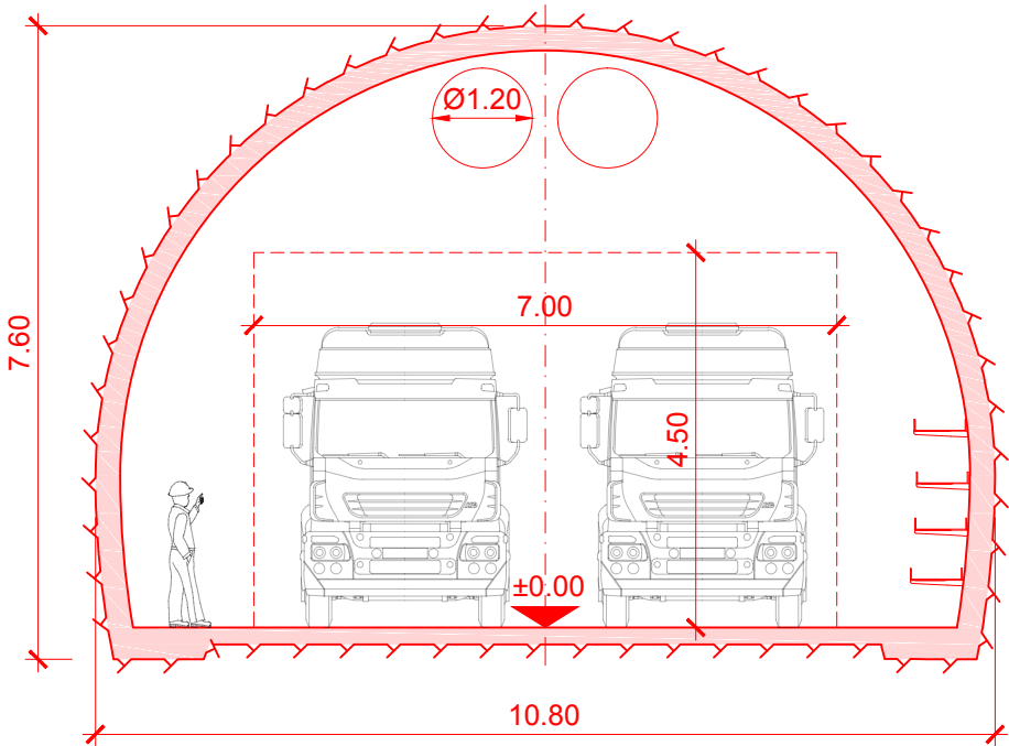
Sección C-C Zona de tránsito central
