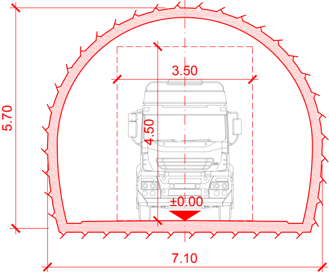
Sección A'-A' Galería de salida principal
