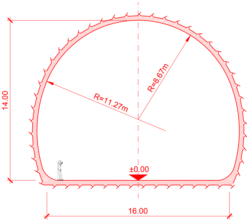
Sección Y-Y Caverna secundaria A=233 m 2
