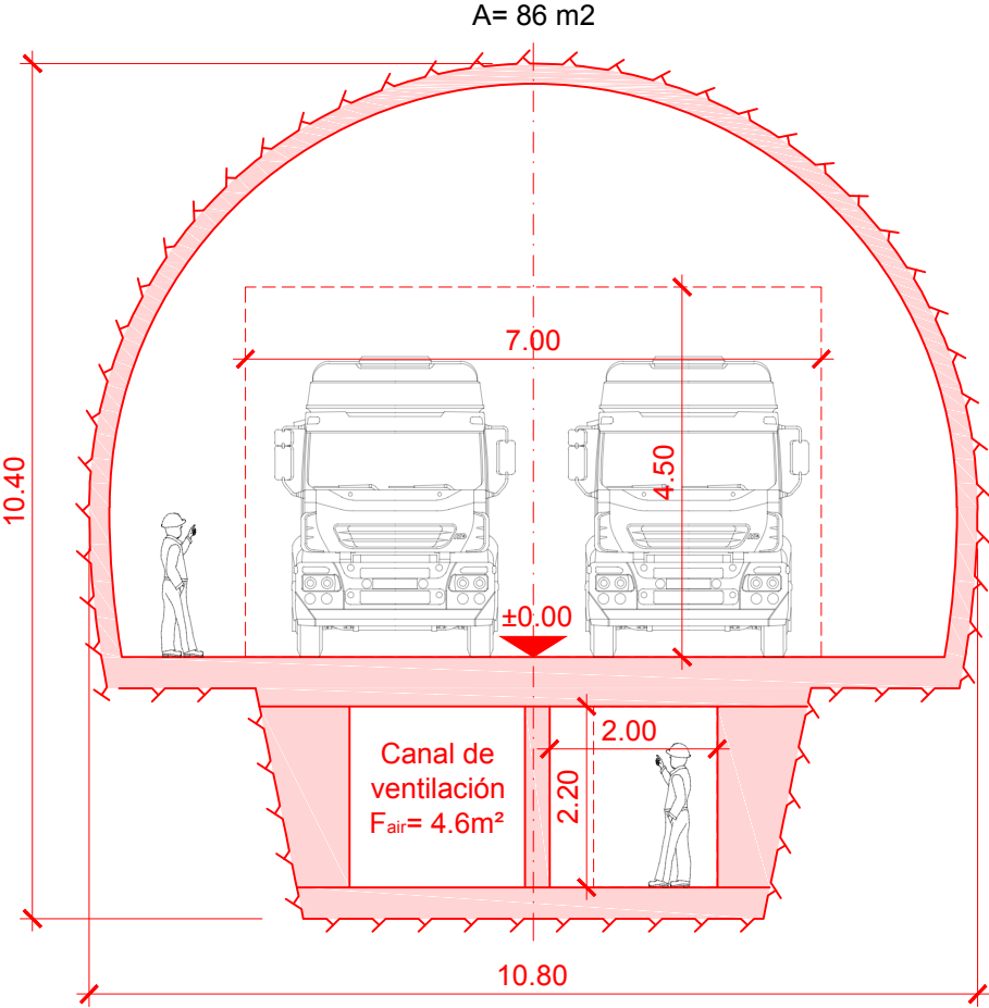
Sección C-C Galería de acceso al fondo del pozo
