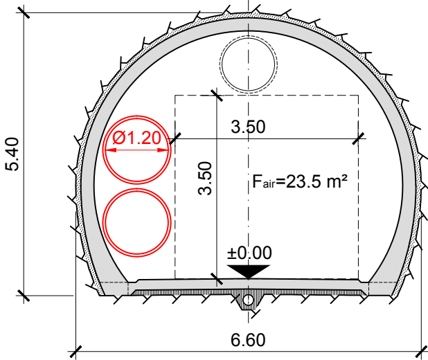
Sección E-E Galería de ventilación (Proyecto TAN)
