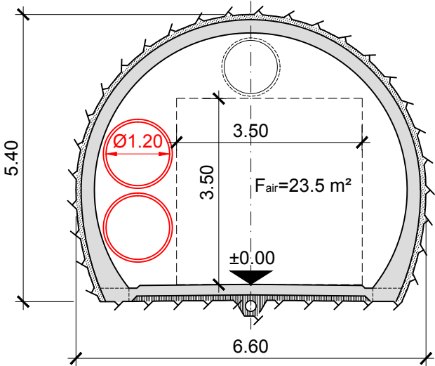
Sección C-C Zona de tránsito central
