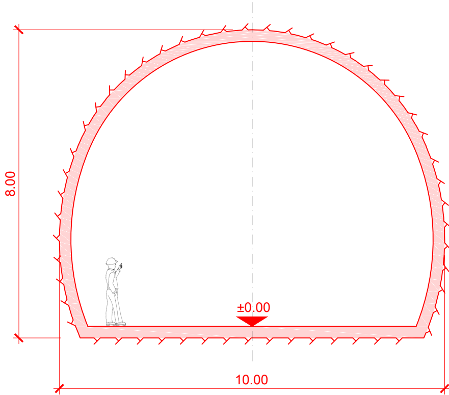
Sección V-V Sala de emergencia/oficina/comedor Sala técnica Sala limpia A=68 m²
