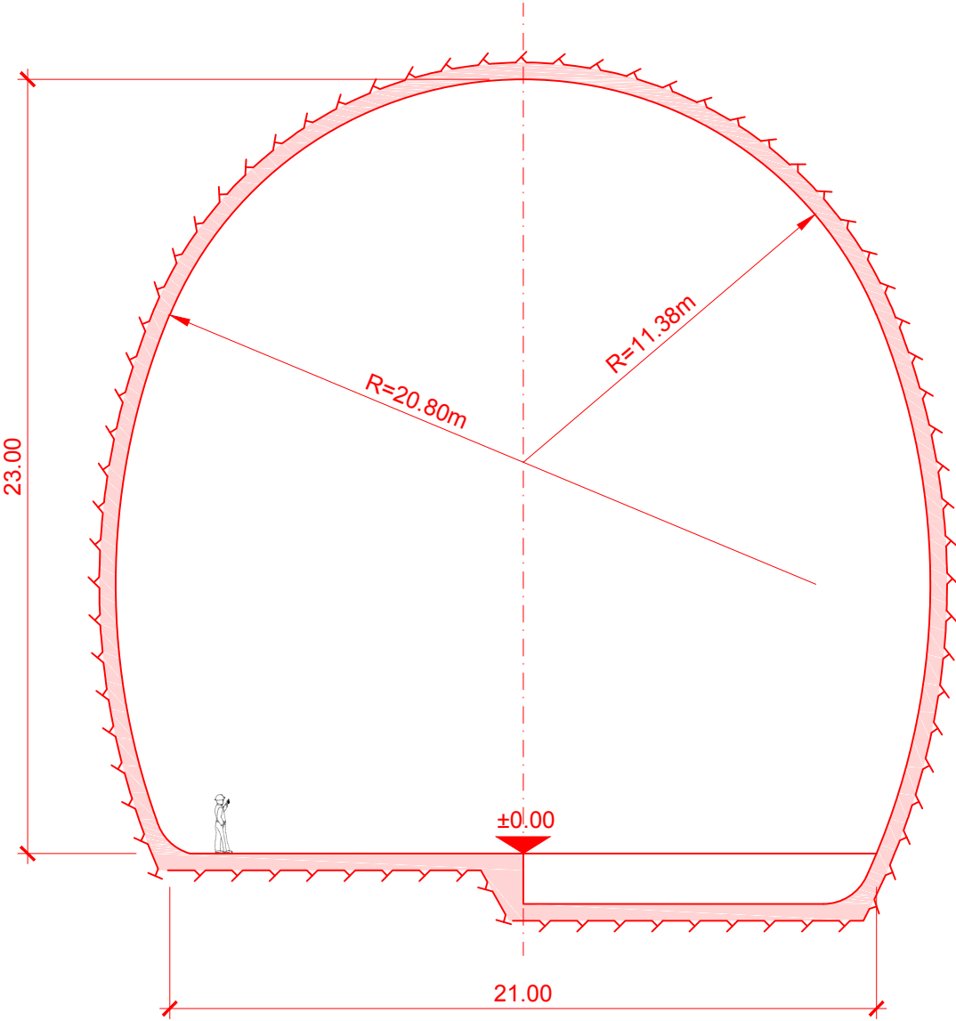
Sección X-X Caverna principal A=530 m 2
