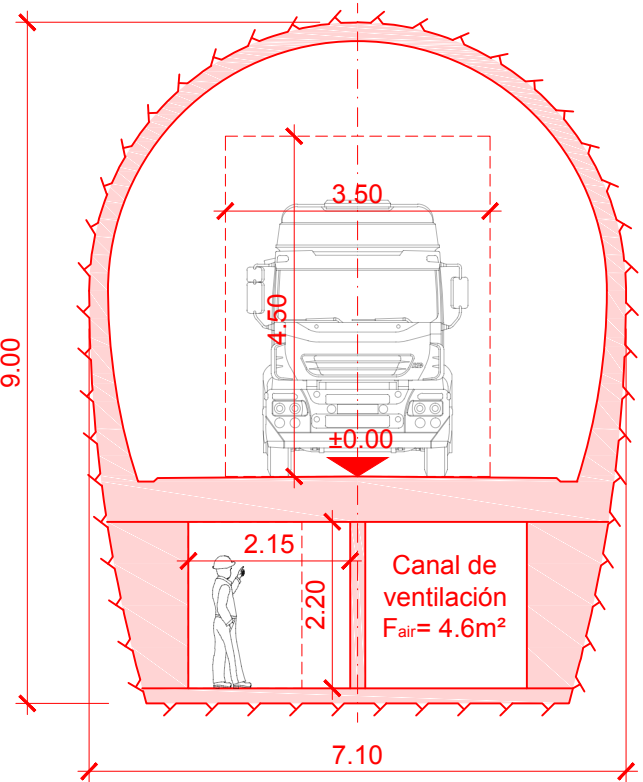
Sección E-E Galería de acceso al fondo del pozo
