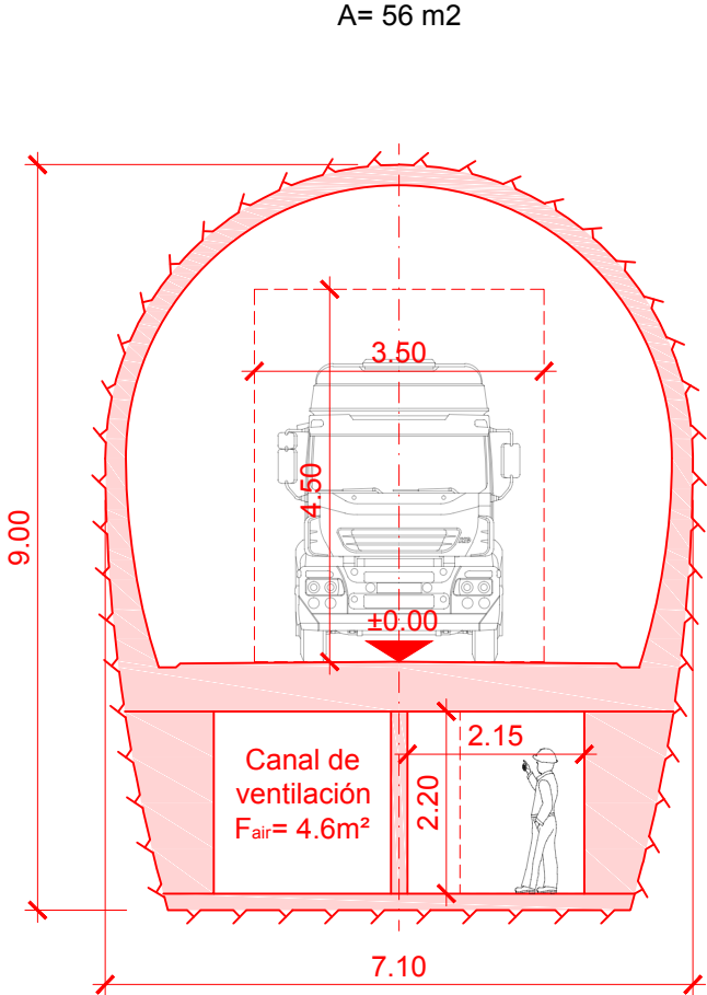
Sección D-D Galería de interconexión vehicular (GIV 15)
