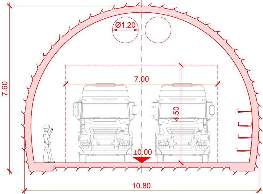
Sección C-C Galería de acceso al fondo del pozo
