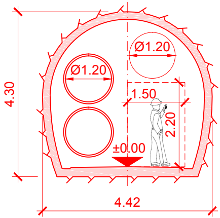
Sección E-E Galería de acceso al fondo del pozo
