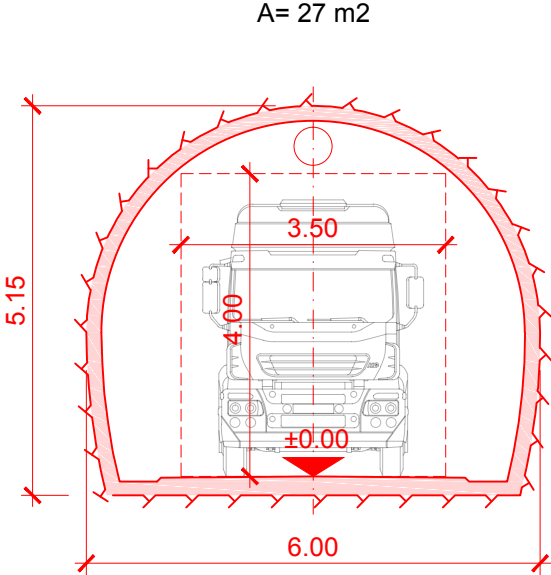
Sección C-C Galería de acceso al fondo del pozo
