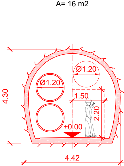
Sección F-F Conexión técnica de ventilación
