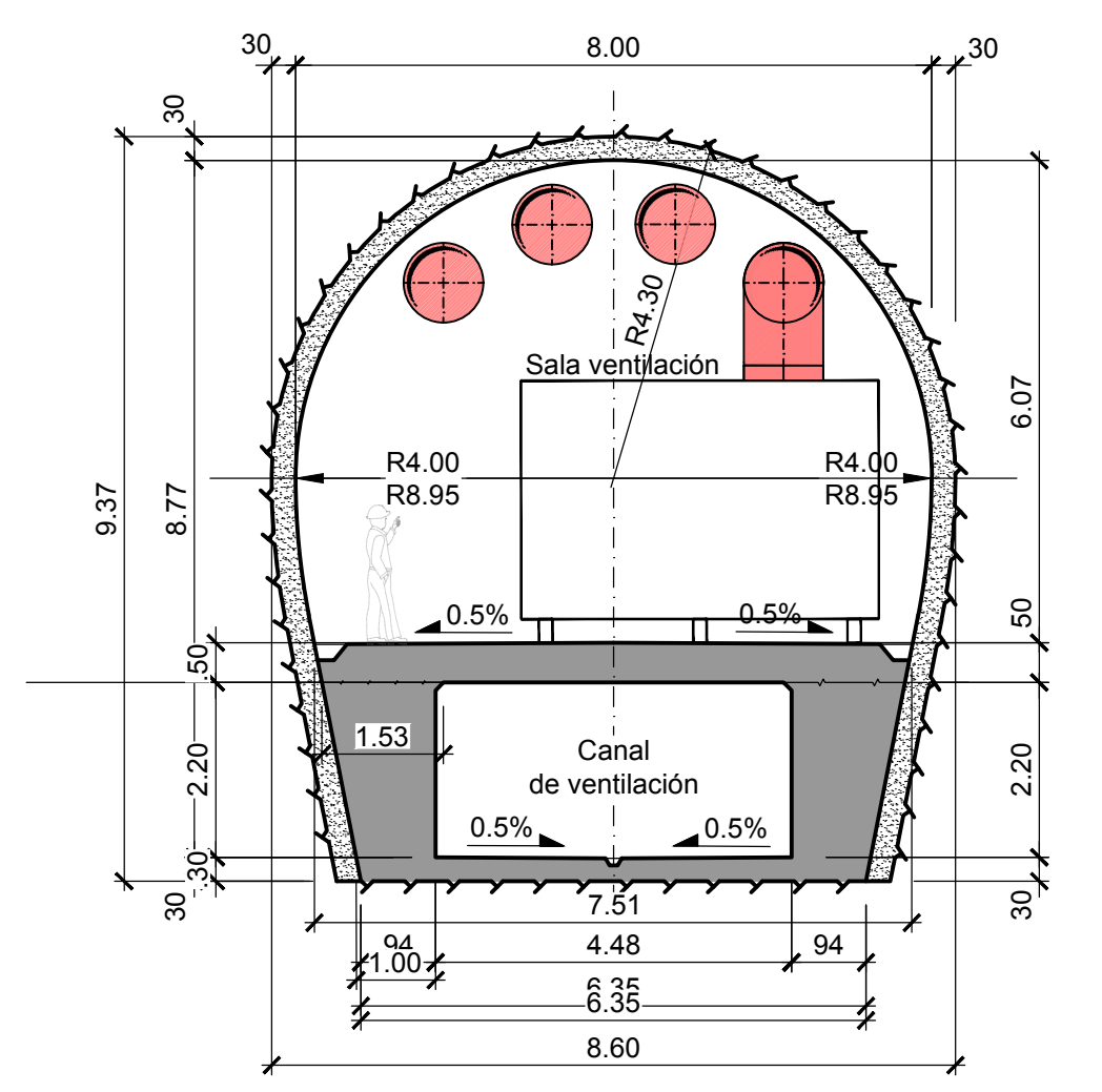
Corte A-A (1:100)
