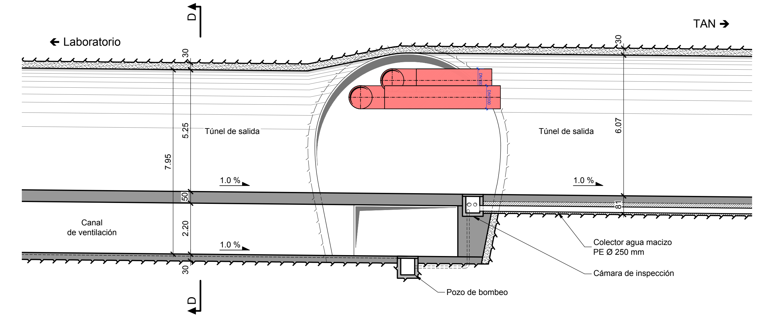
Planta 1-1 (1:100)
