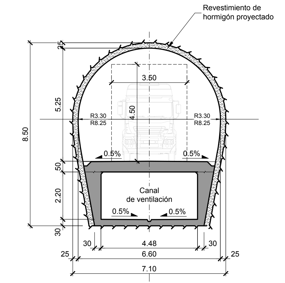
Corte D-D (1:100)
